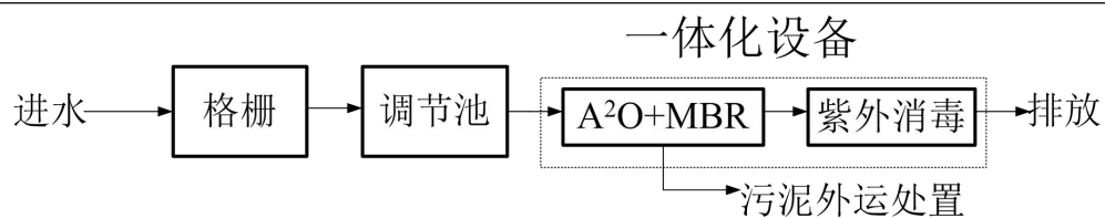
图2-3 污水处理工艺流程图
