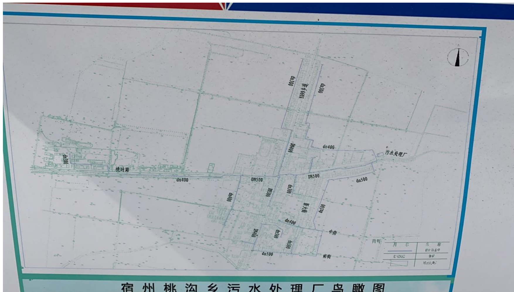
附图三 桃沟乡污水处理厂污水收集管网分布图
