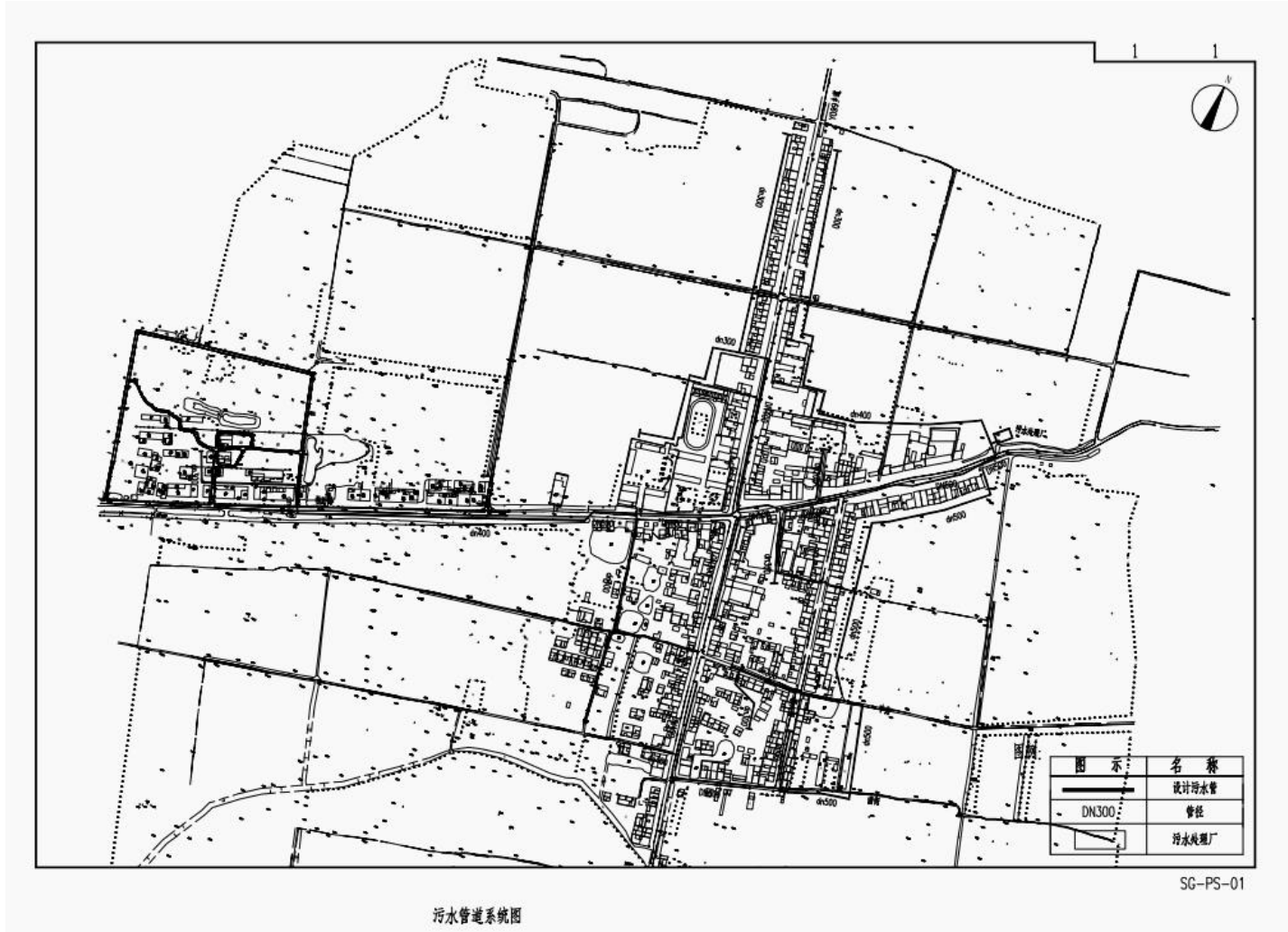
附图四 桃沟乡污水处理厂污水管网施工设计图
