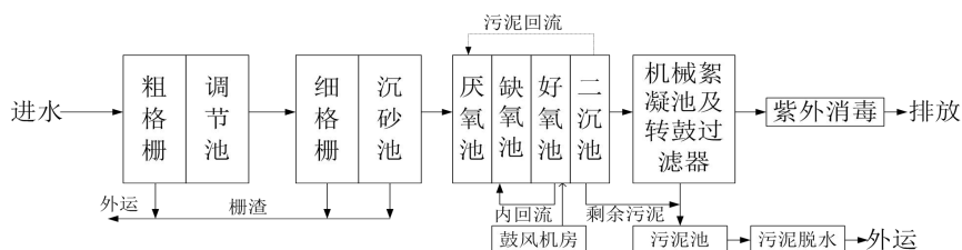
图2-2 污水处理工艺流程图
