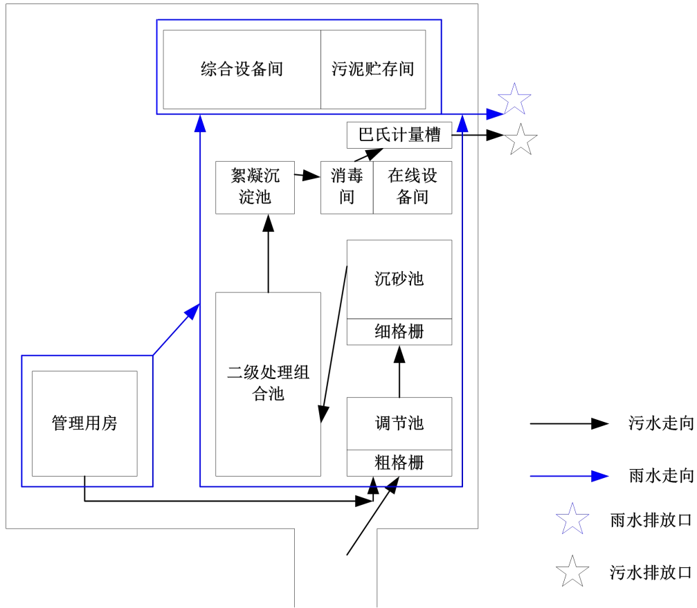
附图2 厂区平面布置图
