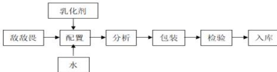
图 3.5-5 敌敌畏产品生产工艺流程图
